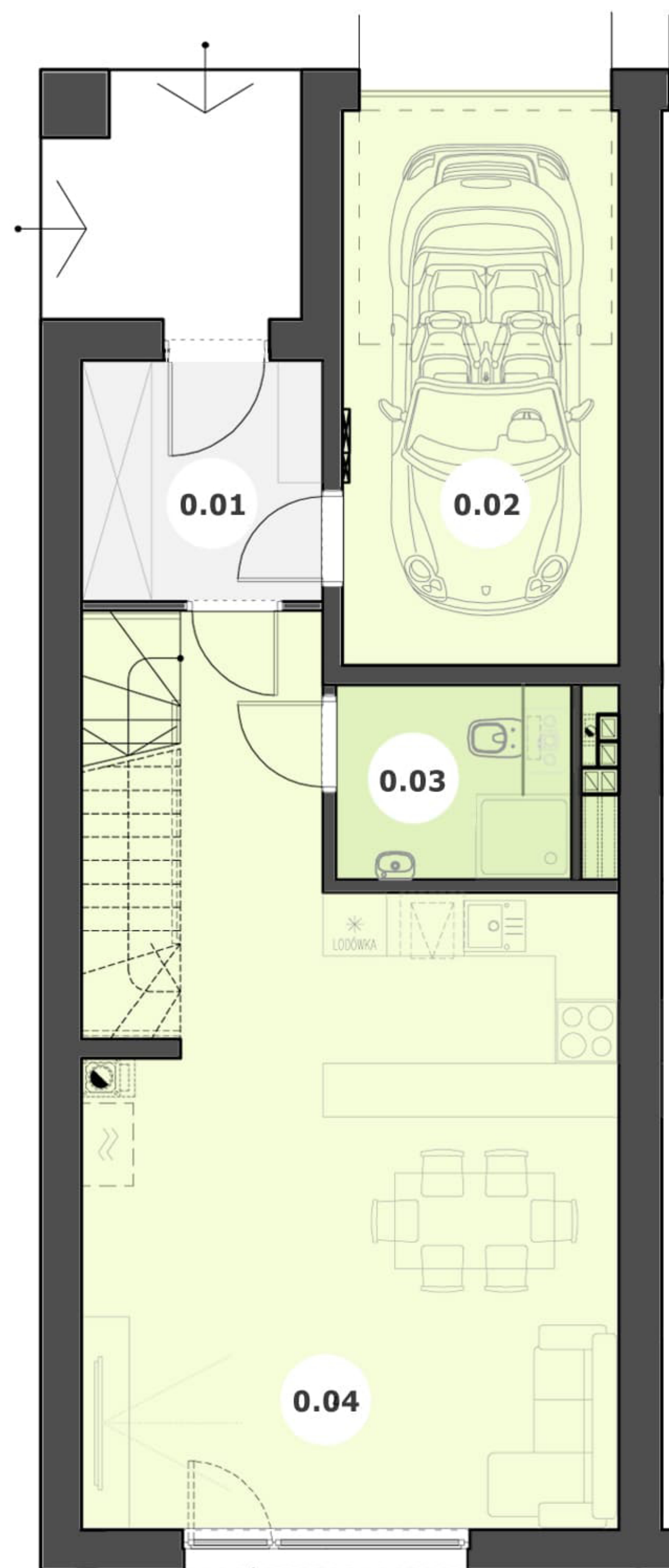
Rzut parteru
